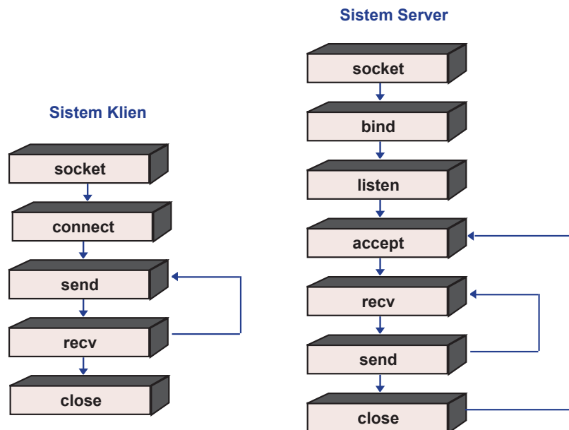
Gambar 3.4 Ilustrasi urutan fungsi socket yang dipanggil oleh client dan server dengan menggunakan paradigma stream.
