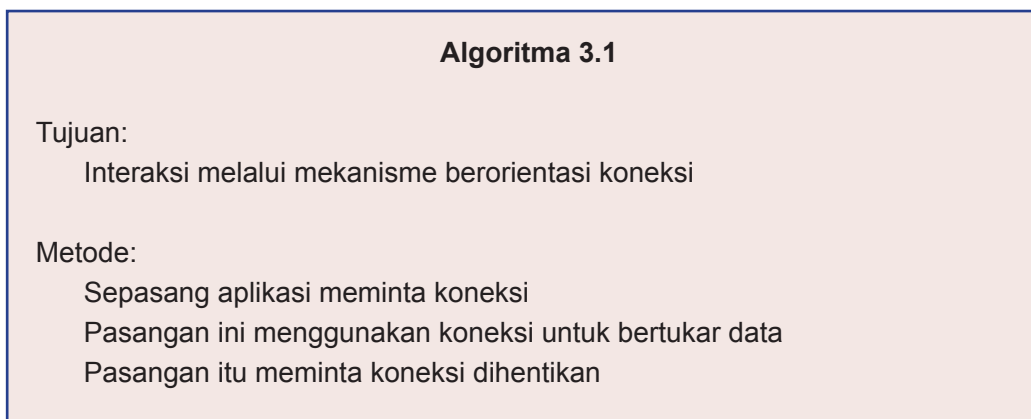
Algoritma 3.1 Komunikasi melalui mekanisme berorientasi koneksi.
