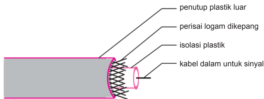
Gambar 7.3 Ilustrasi kabel koaksial dengan pelindung yang mengelilingi kabel sinyal.
