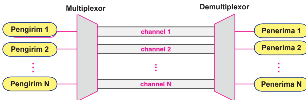
Gambar 11.3 Pandangan konseptual dari Frequency Division Multiplexing (FDM) sebagai penyediaan satu set saluran independen.
