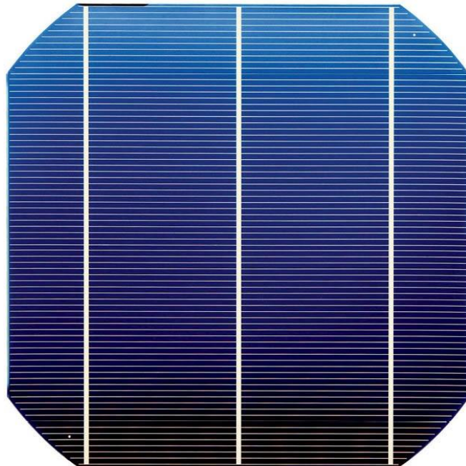
Gambar 3.2 Silikon monokristalin
