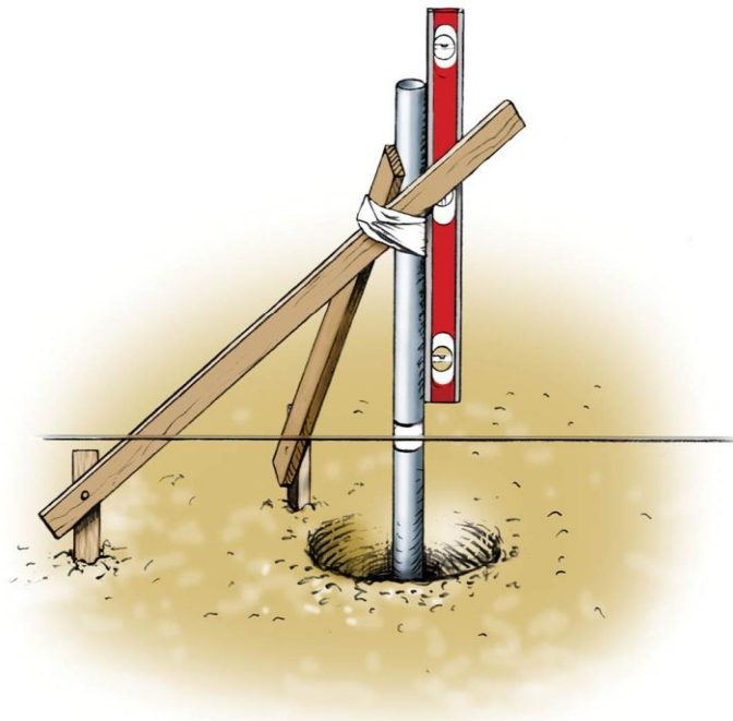
Gambar 7.4 Pengencangan tiang dengan potongan 2x4
